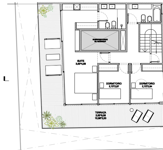
PISO 12º
