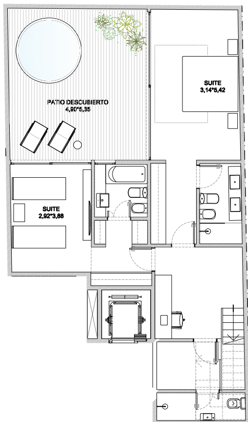
PLANTA BAJA
