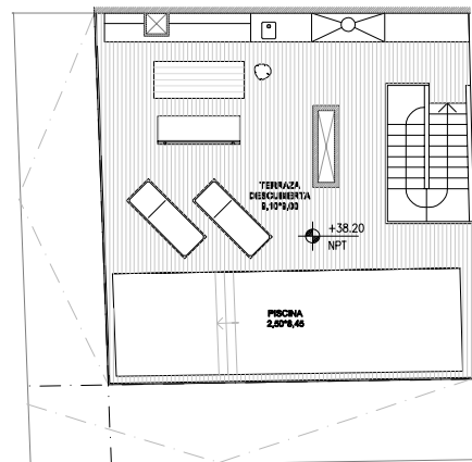
PISO 13º
